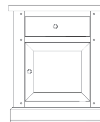
1 Door Cupboard H 840 W 690 D 350
