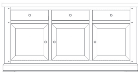
3 Door Sideboard H 915 W 1800 D 490
